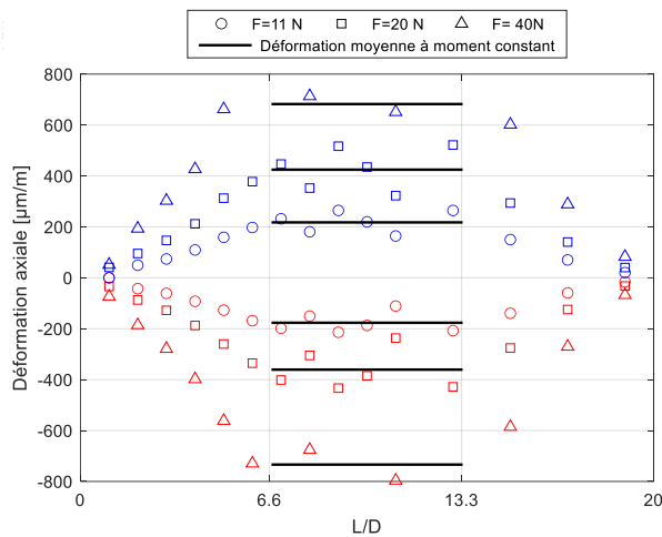
Figure 2. Déformation le long de la longueur du pieu à l'application d'une charge croissante Figure 3. Force par rapport à la déflexion
