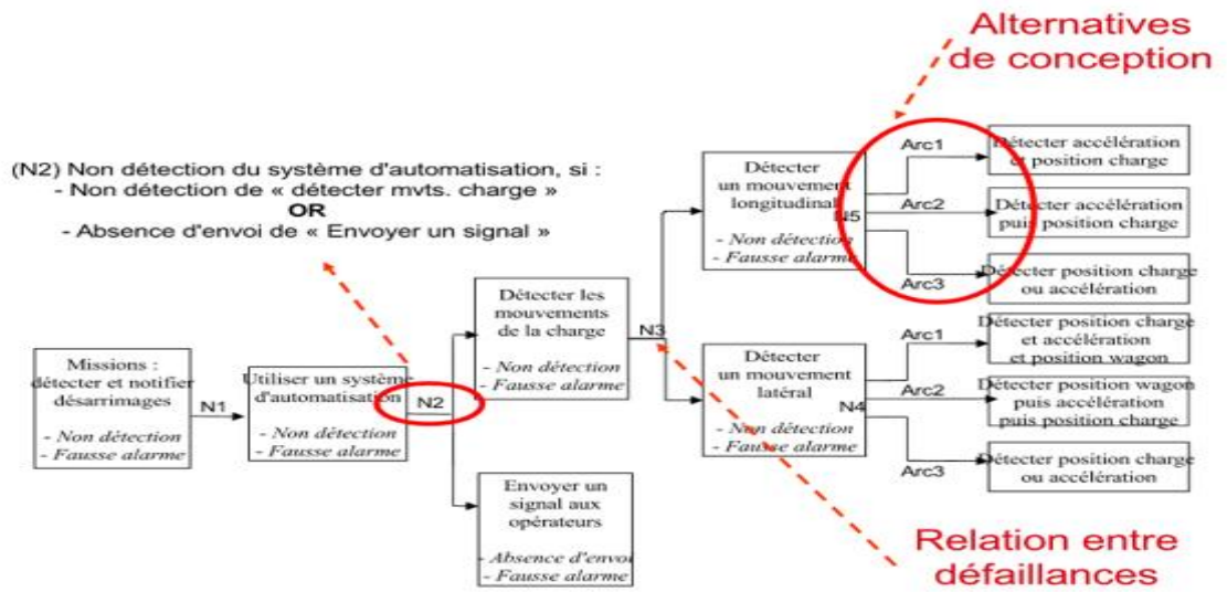
FIGURE 19- APPLICATION À LA SURVEILLANCE DE L'ARRIMAGE DU CAMION
