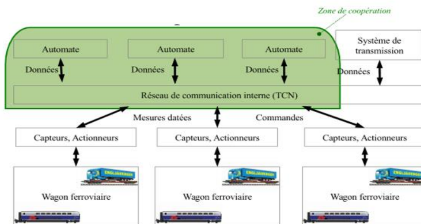
FIGURE 13 : SYSTÈME AUTOMATIQUE POUR UN TRAIN
