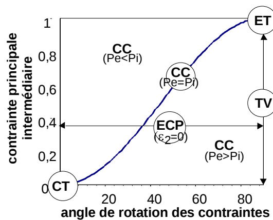
Figure 17. Relations entre les paramètres b et \alpha pour différents appareillages (ECP= essai de cisaillement plan, CC= cylindre creux, CT= compression triaxiale, ET= extension triaxiale, TV= triaxial vrai)
