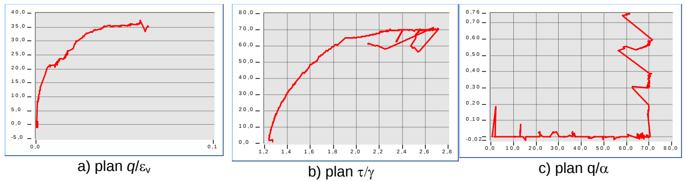
Figure 21. Cisaillement de l'argile de Guiche (PTCC du LCPC)
