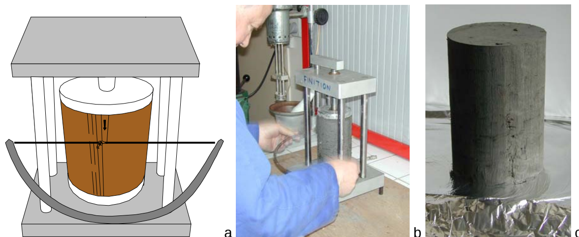
Figure 10. Découpe extérieure d'une éprouvette provenant d'un prélèvement intact
