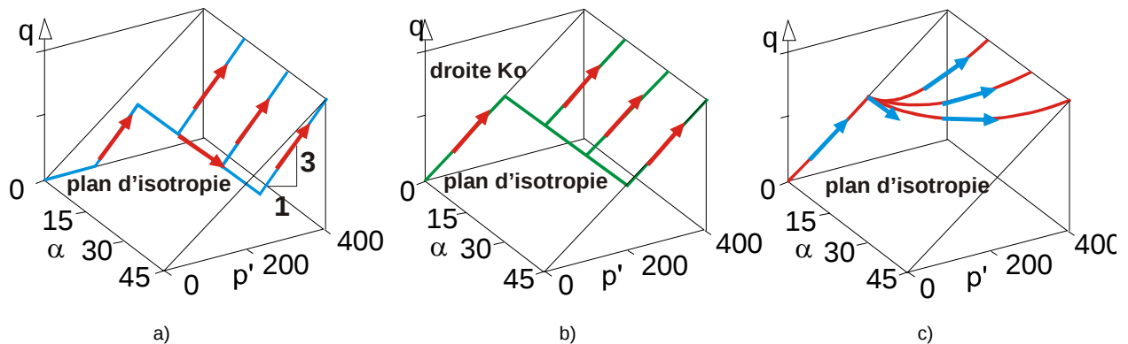
Figure 18. Chemins de contraintes typiques
