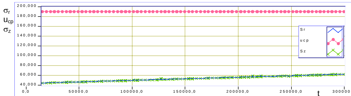
c) Contraintes en fonction du temps
