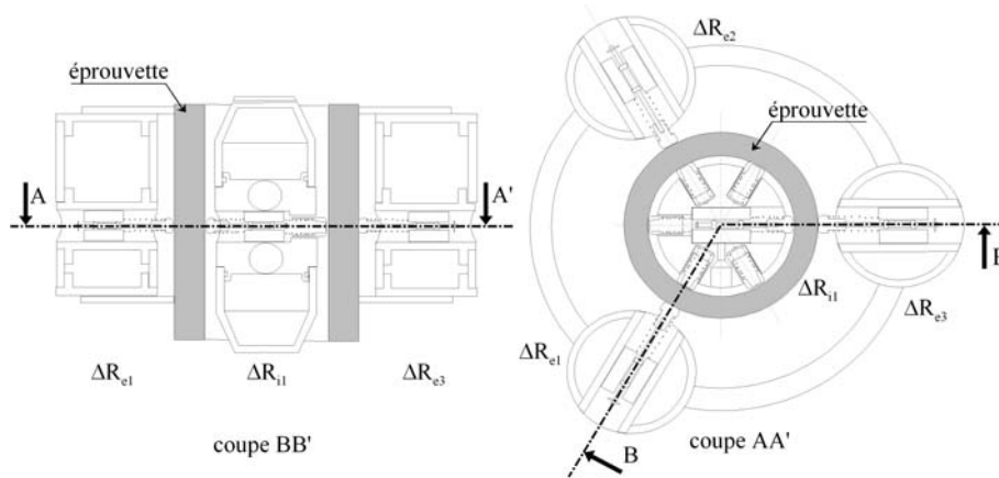
Figure 9. Disposition des capteurs intérieurs et extérieurs (PTCC du LCPC)
