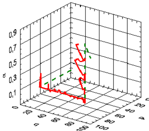
Figure 22. Cisaillement de l'argile de Guiche dans l'espace p, q, \alpha (PTCC du LCPC)
