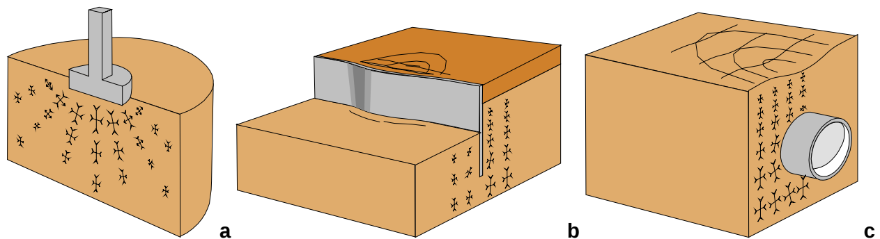
Figure 1. Rotation des contraintes dans les massifs de sol :
