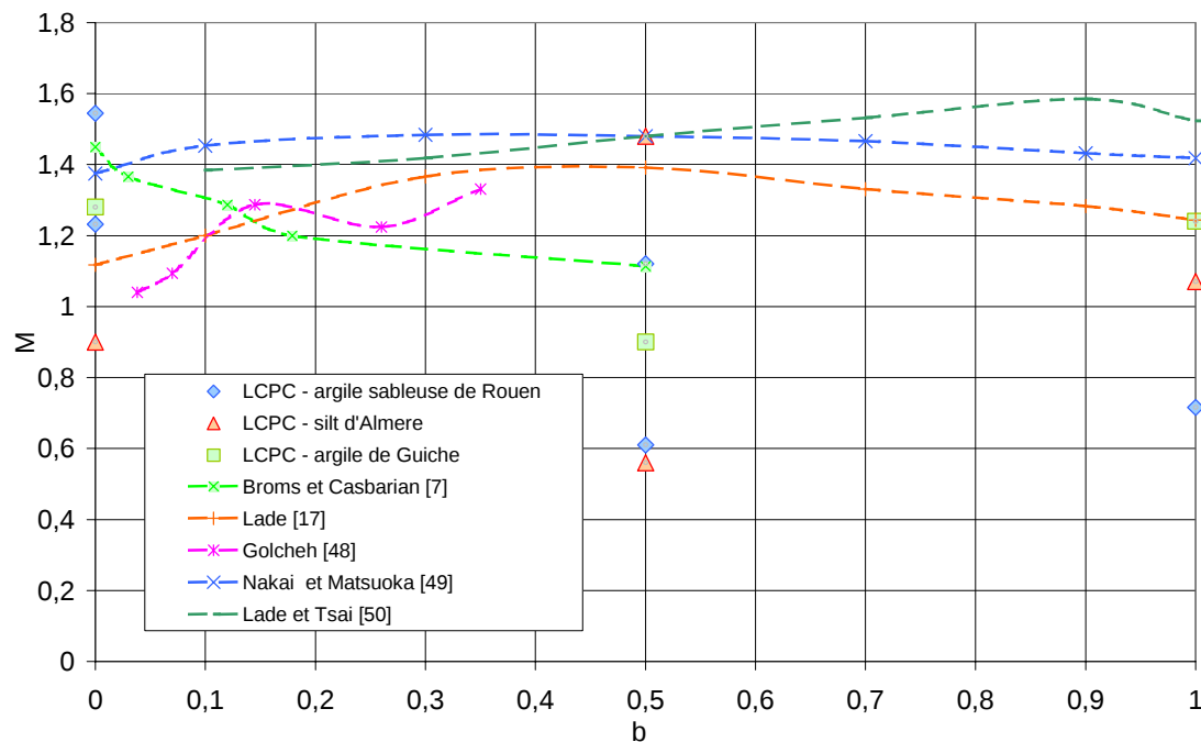
Figure 25. Comparaison des résultats obtenus avec les données de la littérature
