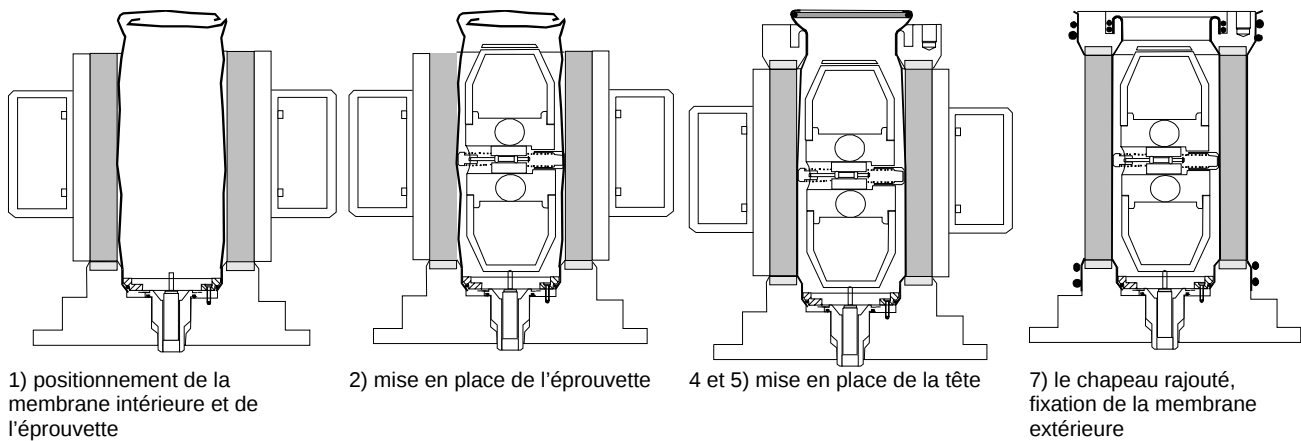
Figure 15. Procédure pour le montage de l'éprouvette
