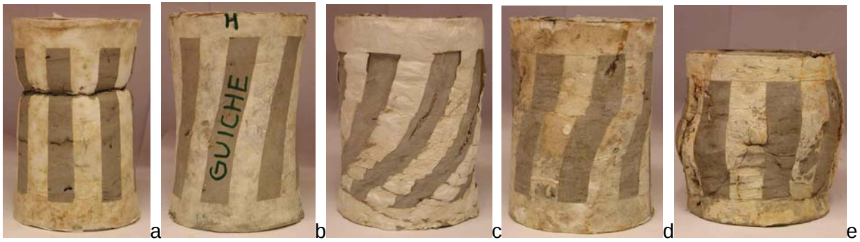
Figure 23. Exemples de modes de rupture obtenus pour l'argile de Guiche : a) extension ; b) extension et cisaillement ; c) cisaillement ; d) cisaillement et compression ; e) compression (PTCC du LCPC)
