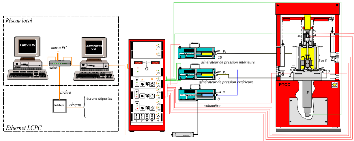
Figure 6. Schéma fonctionnel de la presse triaxiale pour éprouvettes cylindriques creuses (PTCC) du LCPC
