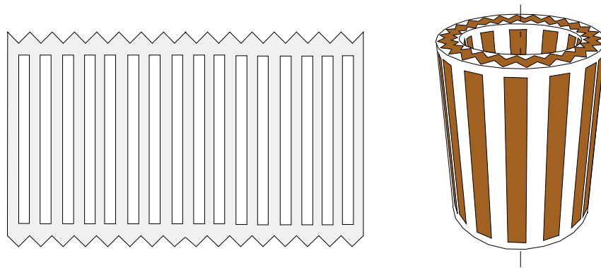
Figure 14. Mise en place du drain latéral ajouré sur l'éprouvette
