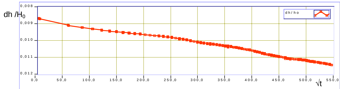
a) Déformation verticale \Delta h/h_0 en fonction de la racine du temps
