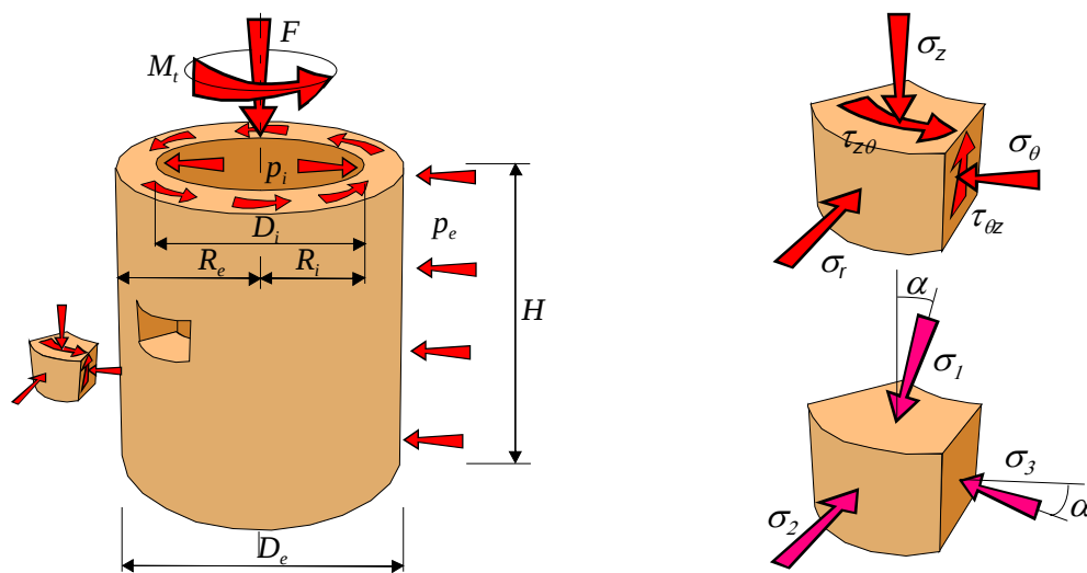
Figure 2. Rotation des contraintes dans une éprouvette cylindrique creuse
