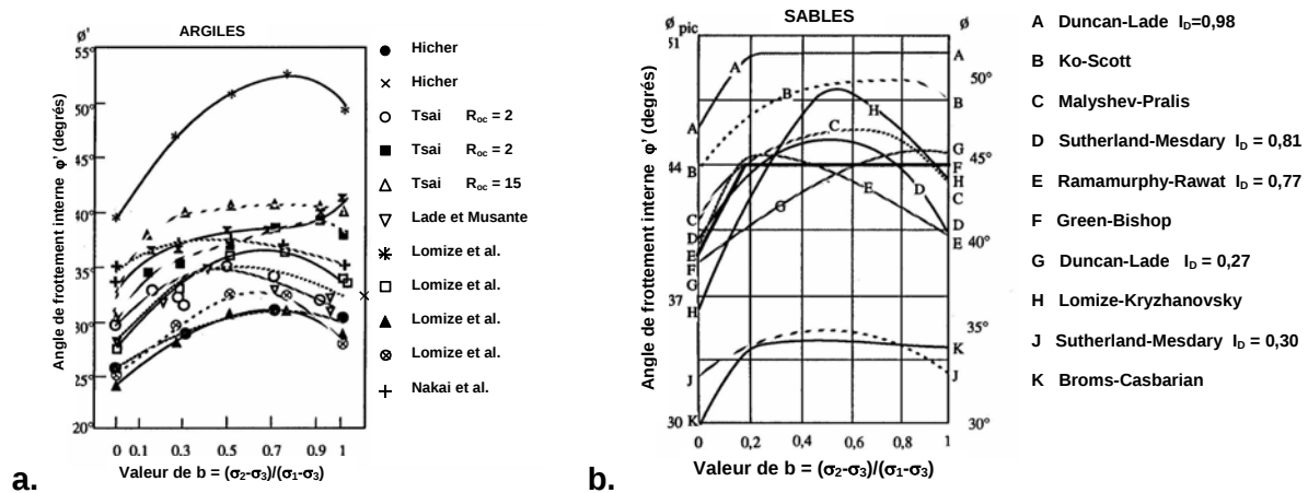
Figure 24. Valeurs de l'angle de frottement interne \phi en fonction du paramètre b de la contrainte principale intermédiaire au vrai triaxial et au cylindre creux : a) pour les argiles ; b) pour les sables (d'après Biarez et Hicher [46])
