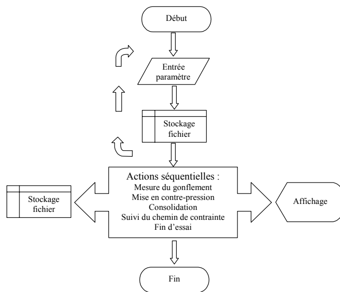
Figure 20. Organigramme général du logiciel du LCPC (PTCC)
