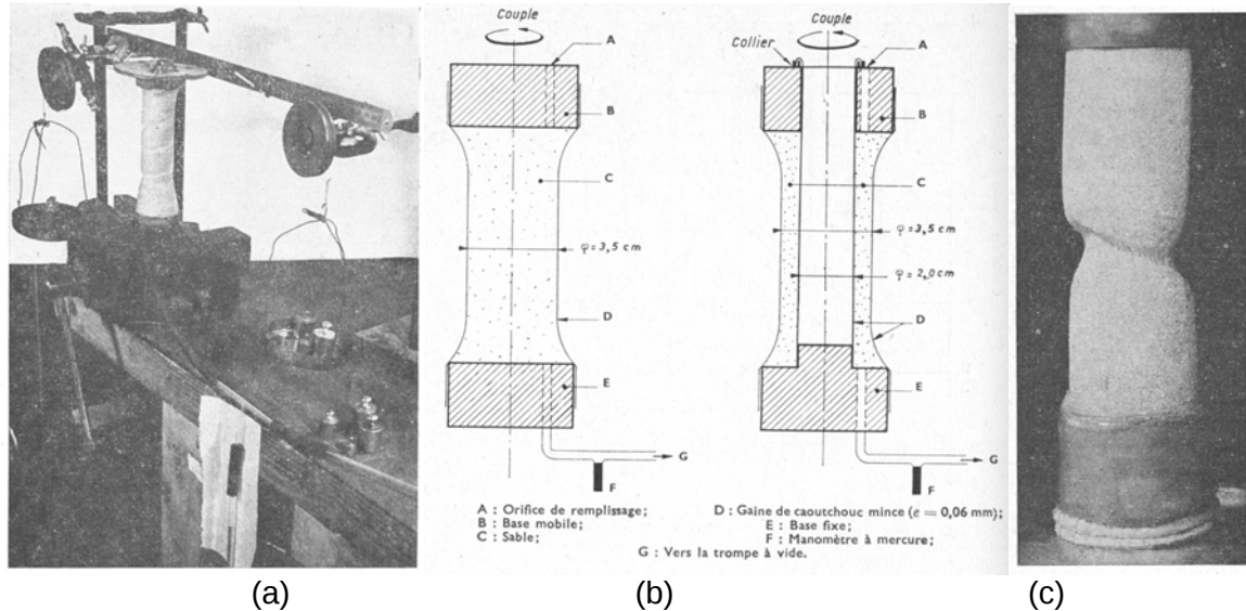
Figure 4. Vue du dispositif en cours d'essai (a), géométrie de l'éprouvette (b) et vue de l'éprouvette après rupture(c) (d'après Habib [13])
