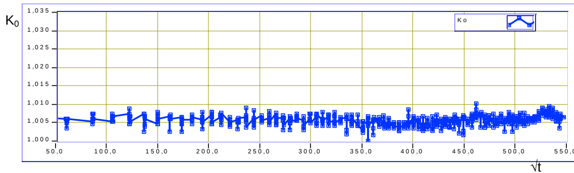
b) Coefficient K_0 en fonction de la racine du temps
