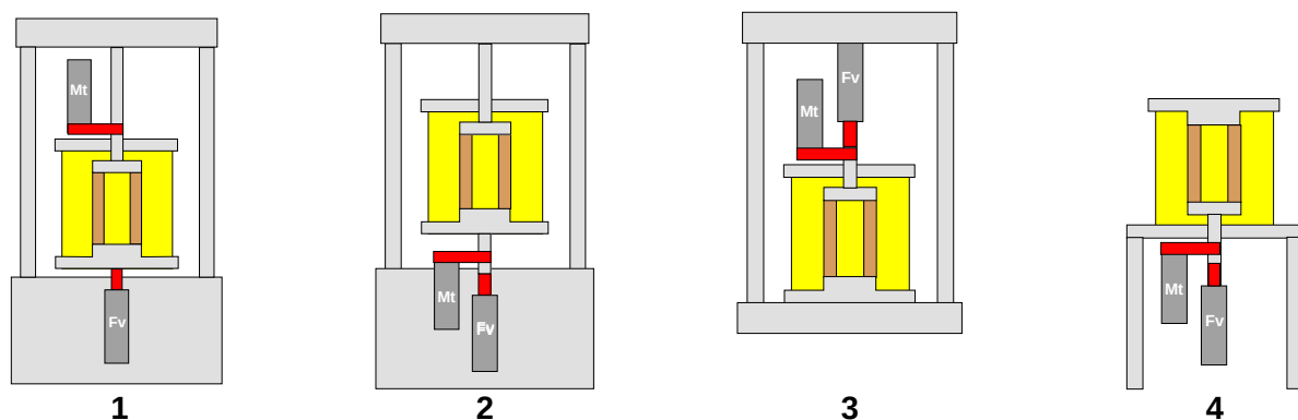
Figure 8. Types de presses triaxiales pour éprouvettes cylindriques creuses
