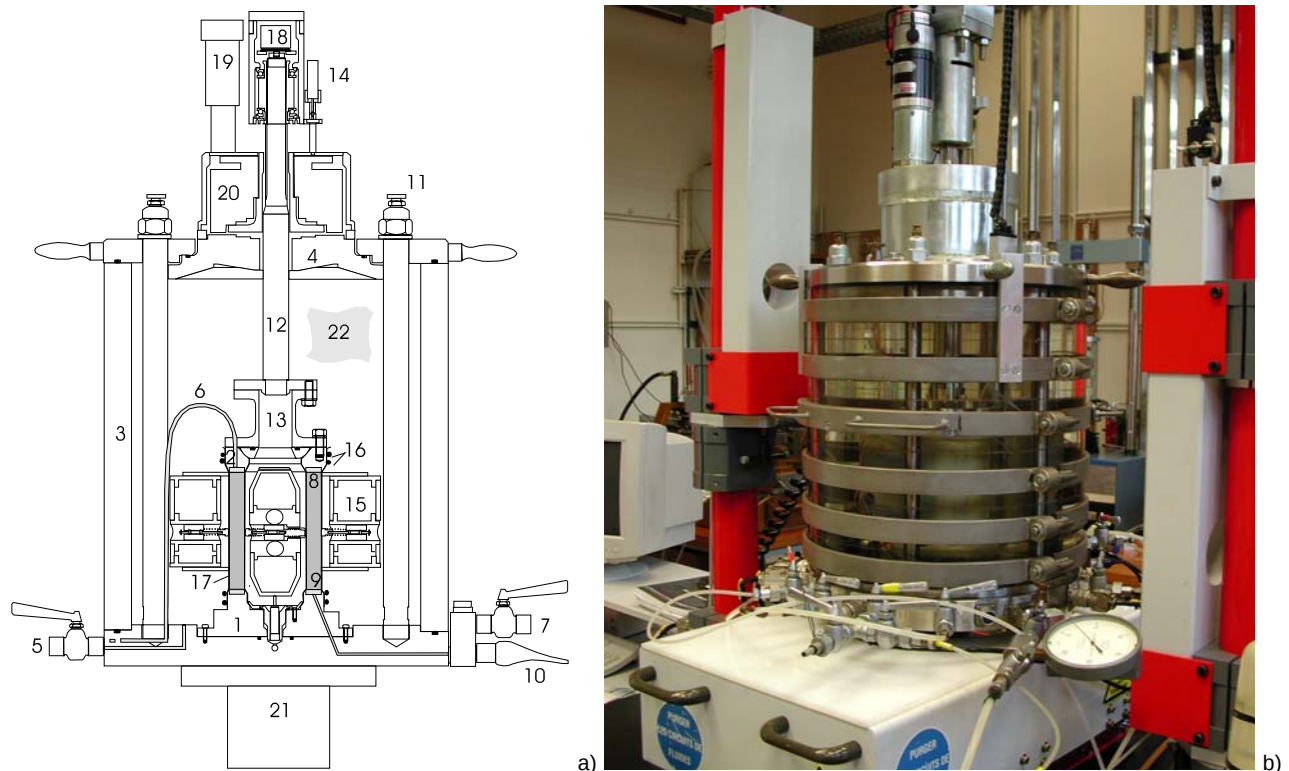
Figure 7. Schéma de la cellule d'essai du LCPC
