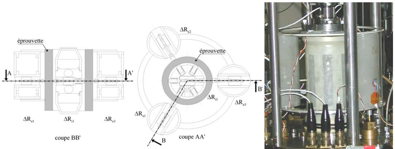
Figure 9. Disposition des capteurs intérieurs et extérieurs (PTCC du LCPC)
