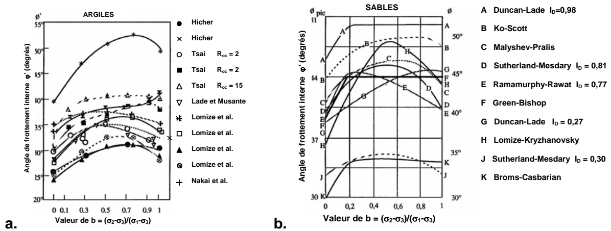
Figure 24. Valeurs de l'angle de frottement interne \varphi en fonction du paramètre b de la contrainte principale intermédiaire au vrai triaxial et au cylindre creux : a) pour les argiles ; b) pour les sables (d'après Biarez et Hicher [46])
