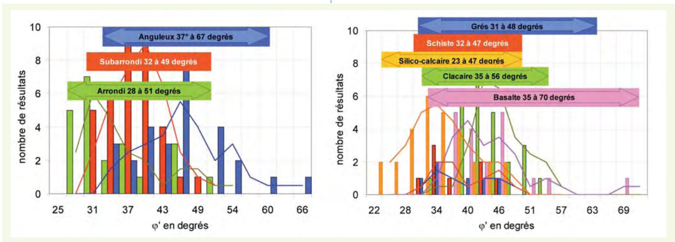
figure 2 Influence de la forme (a) et de la nature (b) des grains sur l'angle de frottement.
