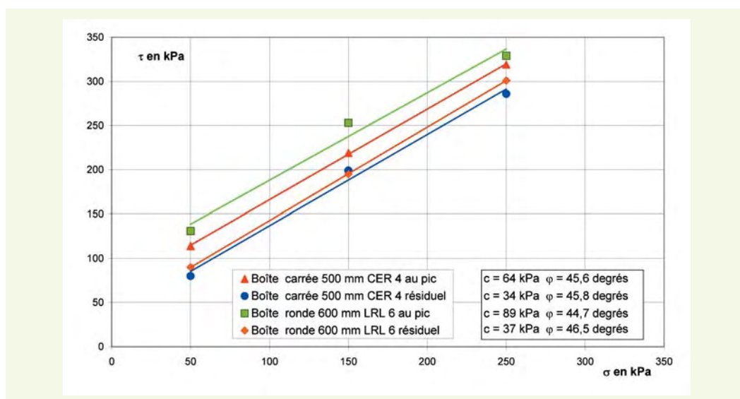
figure 24 Courbes intrinsèques obtenues pour différents appareillages.
