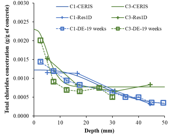
(d) 19 weeks – total chlorides
