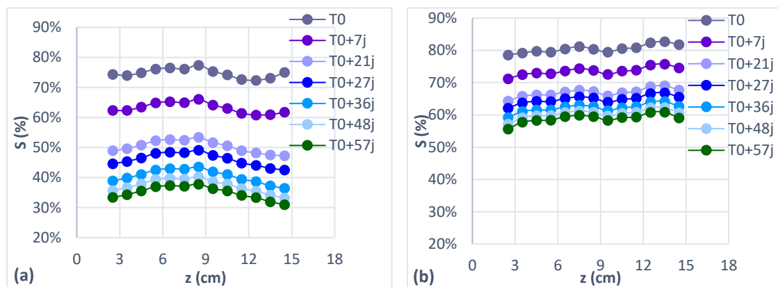
FIGURE 4. Profils de degré de saturation en fonction de la profondeur obtenus pour les deux bétons pendant le séchage – a) Béton C100-0, b) Béton C50-50
